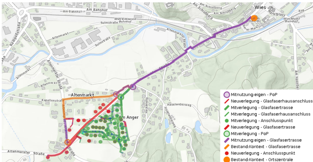
(Plandarstellung)
